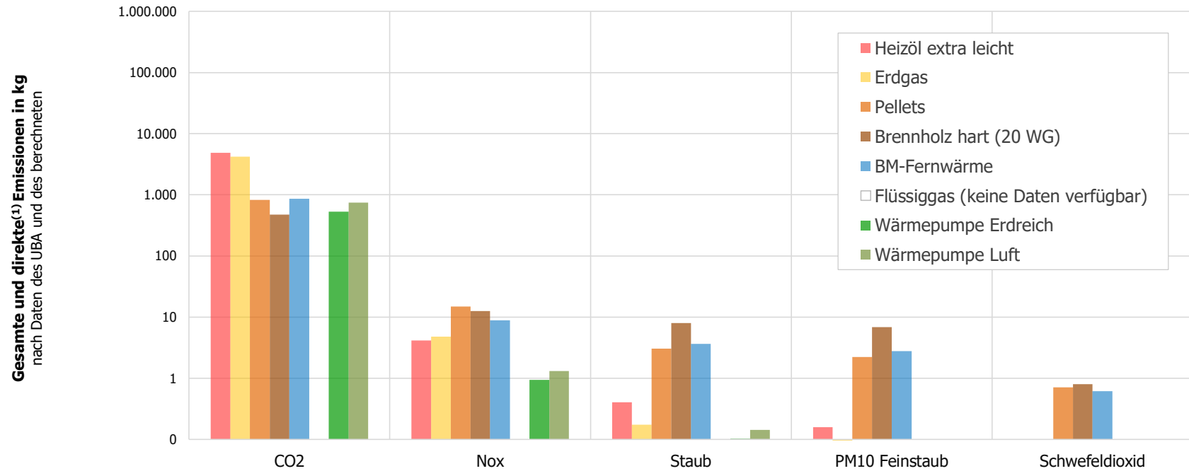
Quelle: Umweltbundesamt 2014 - Emissionsfaktoren unterschiedlicher Heizungssysteme
